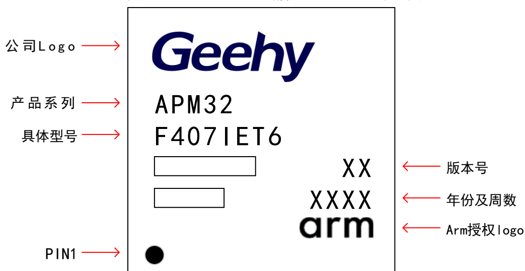
图 19 LQFP176 -176 引脚，24 x24 mm 示意图
